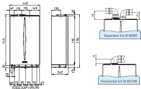
EOLO Extra 24 kW
