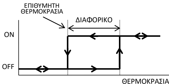
Εικόνα 3- Λειτουργία ψύξης
