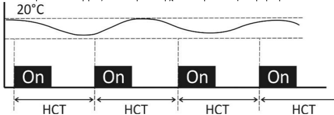
Εικόνα 5- Λειτουργία TPI
