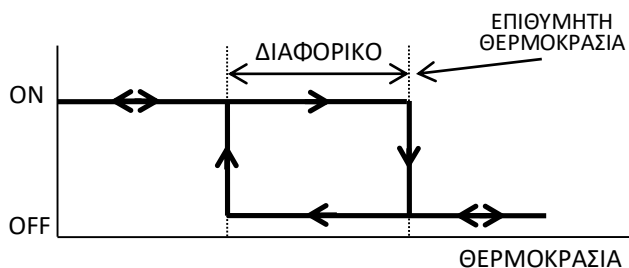
Εικόνα 2- Λειτουργία θέρμανσης
